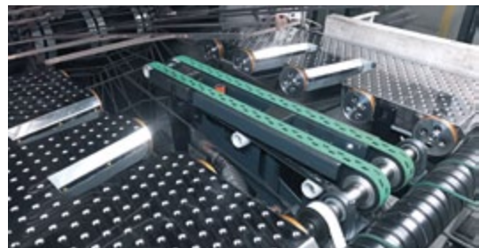
Venturi-Luftdüsen für Tafeltransport mit minimaler Berührung
