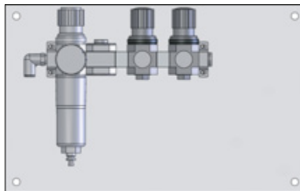
Pneumatikeinheit mit zwei Druckreglern
